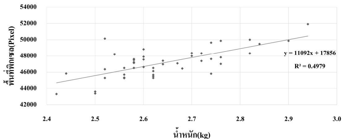
ภาพที่ 9 กราฟความสัมพันธ์ระหว่างน้ำหนักแตงโมและขนาดของพื้นที่จำนวนพิกเซลจากการประมวลผลทางภาพ
