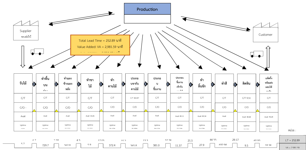
ภาพที่ 5 แผนผังสายธารคุณค่าของกระบวนการผลิต กรณีศึกษาโรงงานผลิตเฟอร์นิเจอร์ไม้ ในสถานการณ์ก่อนปรับปรุง
