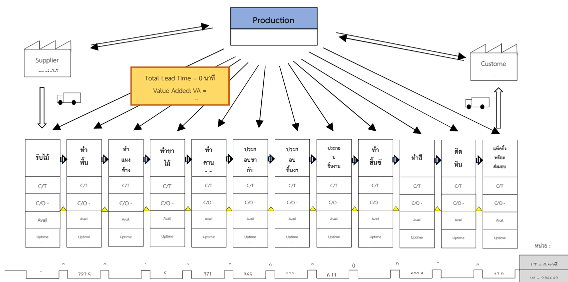
ภาพที่ 10 แผนผังสายธารคุณค่าของกระบวนการผลิต กรณีศึกษาโรงงานผลิตเฟอร์นิเจอร์ไม้ ในสถานการณ์หลังปรับปรุง
