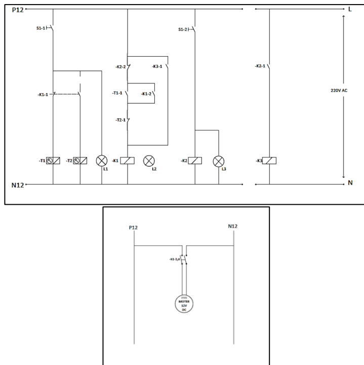
ภาพที่ 4 วงจรควบคุมการเปิด-ปิดมอเตอร์แบบ Manual
