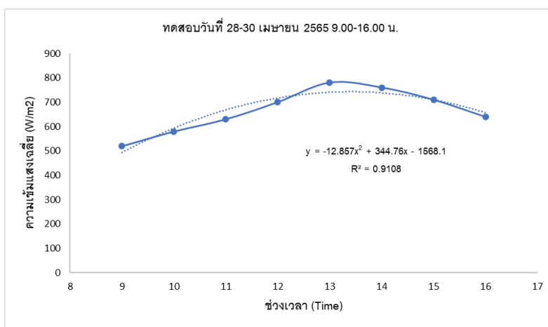
ภาพที่ 9 ความสัมพันธ์ระหว่างความเข้มแสงและช่วงเวลาในการทดสอบ
