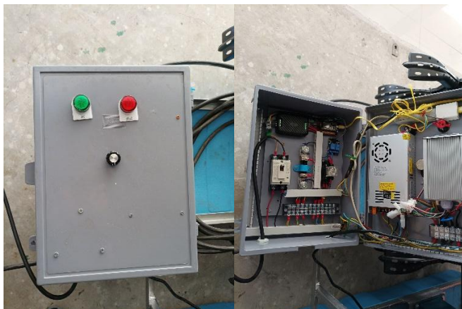
ภาพที่ 5 วงจรควบคุมการเปิด-ปิด มอเตอร์ (ESP 32, 2022) (ETTEAM, 2022)
