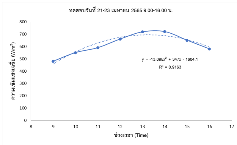
ภาพที่ 7 ความสัมพันธ์ระหว่างความเข้มแสงและช่วงเวลาในการทดสอบ
