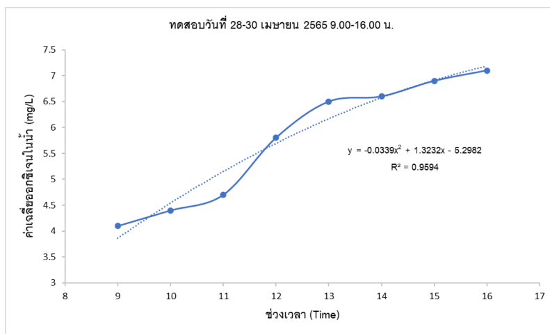
ภาพที่ 8 ความสัมพันธ์ระหว่างค่าออกซิเจนในน้ำและช่วงเวลาในการทดสอบ
