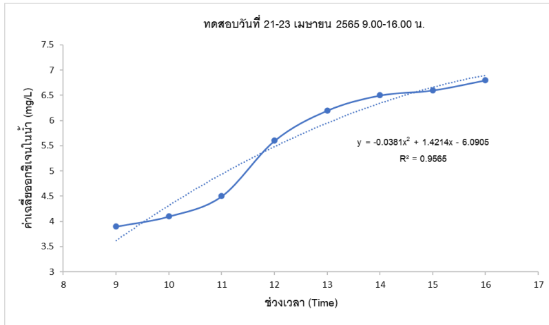
ภาพที่ 6 ความสัมพันธ์ระหว่างค่าออกซิเจนในน้ำและช่วงเวลาในการทดสอบ
