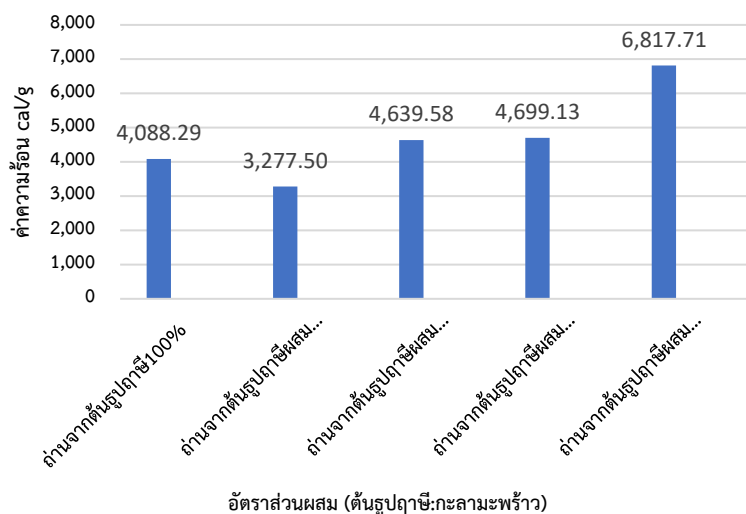
ภาพที่ 11 ค่าความร้อนของถ่านเชื้อเพลิงอัดแท่งจากต้นรูปฤาษีที่อัตราส่วนต่างๆ
