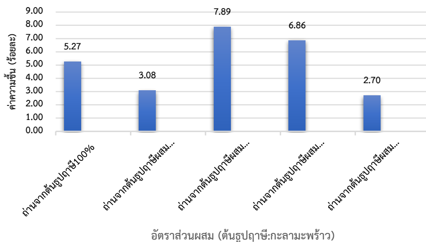
ภาพที่ 10 ค่าความชื้นของถ่านเชื้อเพลิงอัดแท่งจากต้นรูปถั่วที่อัตราส่วนต่างๆ
