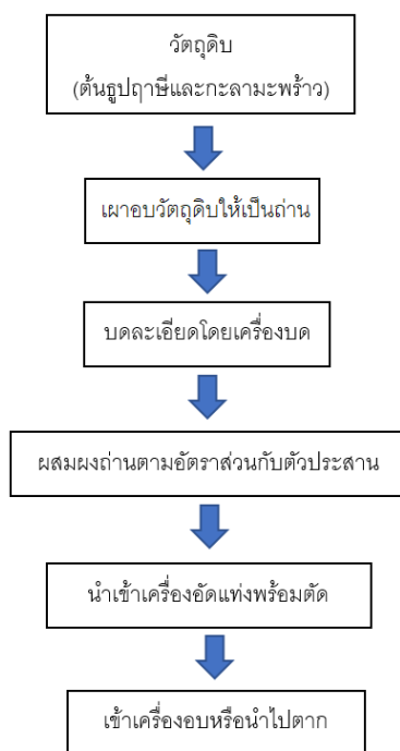
ภาพที่ 1 ขั้นตอนกรรมวิธีการผลิตถ่านอัดแท่งชีวมวลต้นธูปฤๅษี
