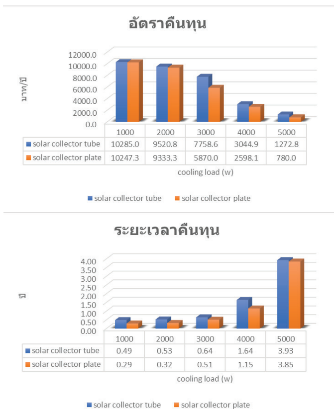
ภาพที่ 7 การประหยัดค่าใช้จ่ายไฟฟ้าที่ลดลงและระยะคืนทุนของระบบปรับอากาศแบบแยกส่วนร่วมกับตัวเก็บรังสีแสงอาทิตย์
