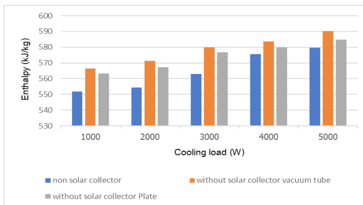
ภาพที่ 4 เอนทัลปีสารทำความเย็นก่อนเข้าคอนเดนเซอร์เทียบกับภาระการทำความเย็น ที่อุณหภูมิห้อง ปรับอากาศ 25°C
