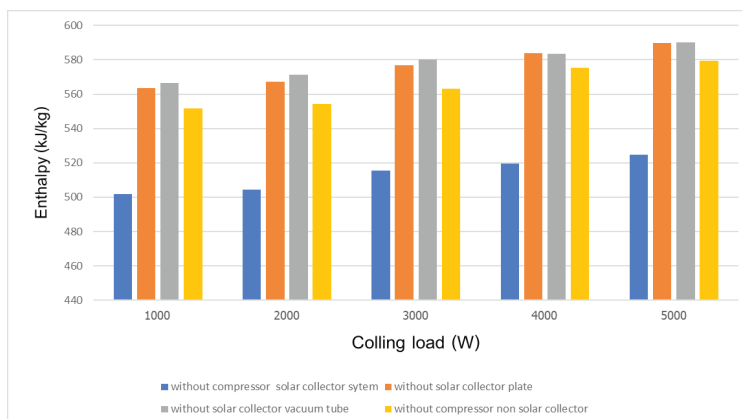
ภาพที่ 5 การเปลี่ยนแปลงของเอนทัลปีของสารทำความเย็นที่ออกจากคอมเพรสเซอร์กับตัวเก็บรังสีแสงอาทิตย์ เทียบกับภาระการทำความเย็นที่อุณหภูมิห้องปรับอากาศ 25°C
