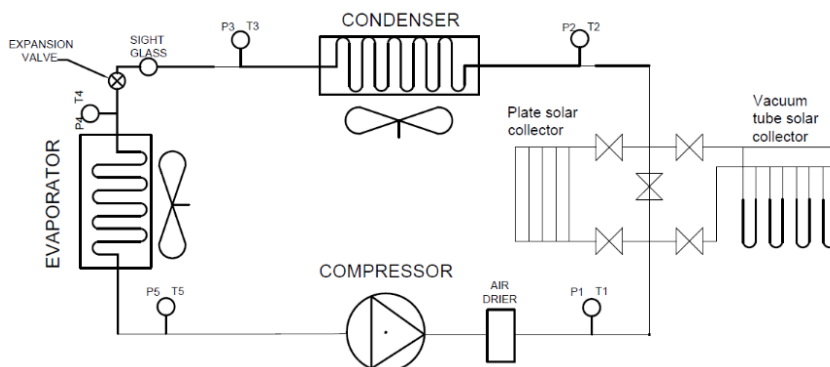
ภาพที่ 1 ระบบปรับอากาศแบบแยกส่วนชนิดอัดไอร่วมกับตัวเก็บรังสีแสงอาทิตย์
