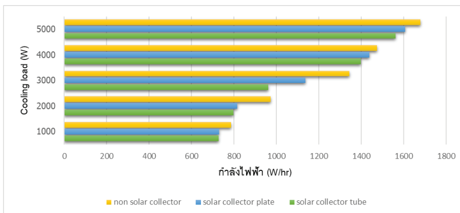
ภาพที่ 6 ค่ากำลังไฟฟ้าเฉลี่ยต่อชั่วโมงเทียบกับภาระการทำความเย็นของห้องปรับอากาศที่ 25°C
