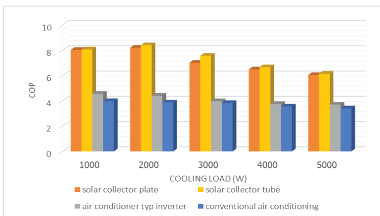
ภาพที่ 2 ค่าสัมประสิทธิ์ของสมรรถนะเทียบกับภาระการทำความเย็น ที่อุณหภูมิ 25^\circ\text{C}
