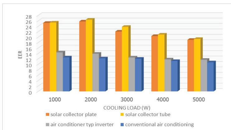
ภาพที่ 3 ค่าอัตราส่วนประสิทธิภาพพลังงานเทียบกับภาระการทำความเย็น ที่อุณหภูมิ 25^\circ\text{C}
