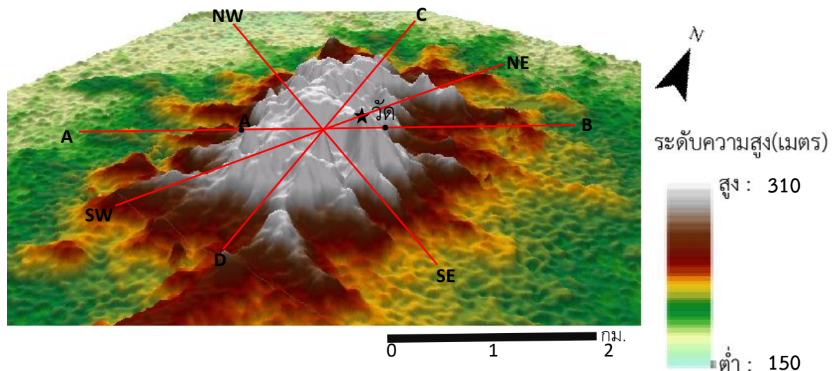
รูป 5 ภาพถ่าย DEM กึ่งสามมิติ (จาก รูป 2ค) แบบมุมมองเฉียง แสดงภูมิลักษณะของภูพระอังคารที่ปรากฏเป็นเนินกลมทรงสูงในบริเวณตอนกลาง เส้นสีแดง 4 เส้นแสดงแนวตัดภูมิประเทศในทิศต่างๆ 4 แนว คือ ทิศเหนือ-ใต้, ทิศตะวันออก-ตก, ทิศตะวันออกเฉียงเหนือ-ตะวันตกเฉียงใต้, และทิศตะวันตกเฉียงเหนือ-ตะวันออกเฉียงใต้ โดยที่ทิศตะวันออกเฉียงเหนือ-ตะวันตกเฉียงใต้ ตัดผ่านวัด
