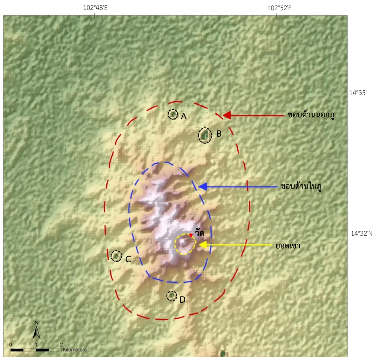
รูป 3ก: ภาพจากดาวเทียม SRTM DEM แสดงขอบด้านในภูเขาไฟ (เส้นปะสีน้ำเงิน, 3 x 4.5 กม.) และขอบด้านนอก (เส้นปะสีแดง, 5 x 8 กม.) รวมทั้งยอดเขา (เส้นปะสีเหลือง) ของภูพระอังคารและวัดเขาพระอังคาร (จุดแดง)[หมายเหตุ : A, B, C และ D คือภาพที่เกิดจากการประมวลผลคลาดเคลื่อน (errors in image processing)]
