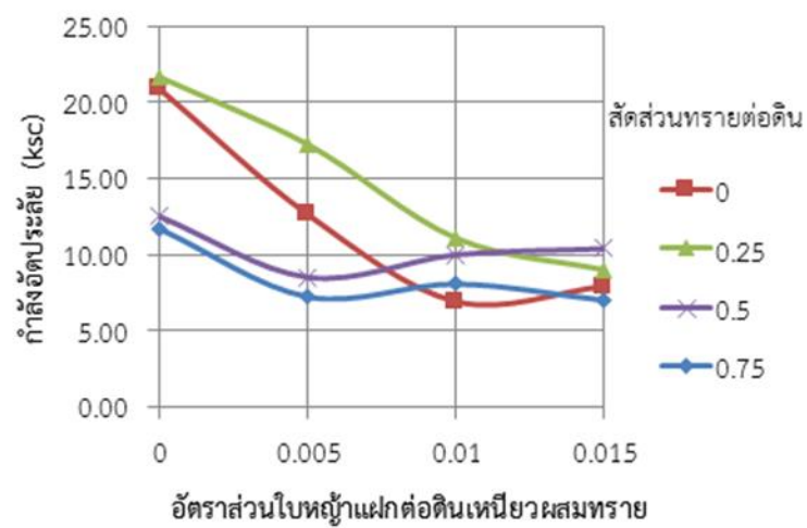
ภาพที่ 8 ความสัมพันธ์ระหว่างกำลังรับแรงอัดของอิฐดินดิบกับปริมาณใบหญ้าแฝก ยาว 4 เซนติเมตร ที่สัดส่วนทรายต่อดินต่าง ๆ
