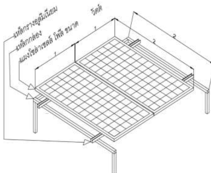
ภาพที่ 2: โครงสร้างแผงโซล่าเซลล์
