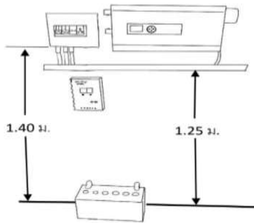
ภาพที่ 1: โครงสร้างและขนาดของชุดสาธิตการติดตั้งโซล่าเซลล์ระบบ ไฮบริด ขนาด 500 วัตต์
