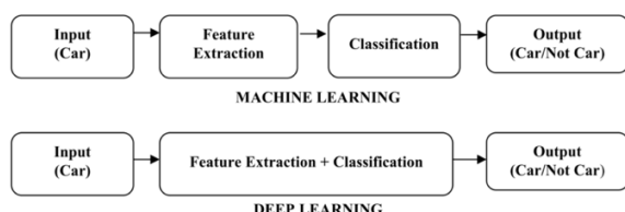
รูปที่ 1 แสดงกระบวนการประมวลผลระหว่างการเรียนรู้ของเครื่องจักรและการเรียนรู้เชิงลึก [2]
