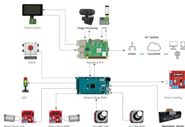
รูปที่ 4 แผนผังการการเชื่อมต่ออุปกรณ์ควบคุมของหุ่นยนต์
