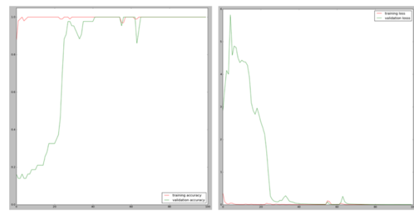
รูปที่ 8 กราฟแสดงความสัมพันธ์ระหว่าง accuracy, loss กับ epochs ของเทคนิค MobileNetV2
