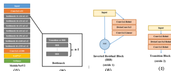
รูปที่ 3 โครงสร้างของ MobileNetV2 (ก) Core block (ข) Bottleneck Block (ค) Inverted (ง) Transition Block
