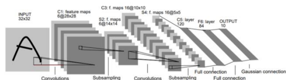
รูปที่ 2 โครงสร้างของโครงข่ายประสาทแบบคอนโวลูชัน [3]
