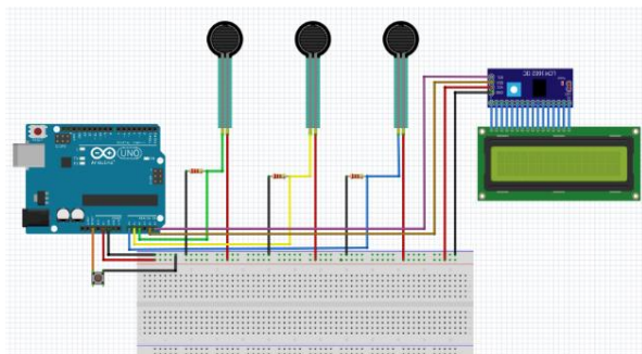
รูปที่ 2 แสดงวงจรของอุปกรณ์ต้นแบบ
