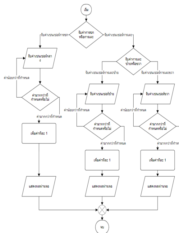
รูปที่ 1 แผนผังการทำงานของระบบ
