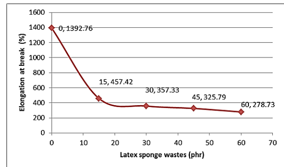
ภาพที่ 10 สมบัติการยืดตัว ณ จุดขาดของยาง STR 5L ที่เติม ฟองน้ำลาเท็กซ์เหลือทิ้ง ที่มีปริมาณต่างๆ
